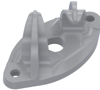
REF : 101759 Intermédiaire alu V3. Tous les 15 mètres maximum. Entraxe : 2 trous 141 mm. Fixation : M10 ou M12
