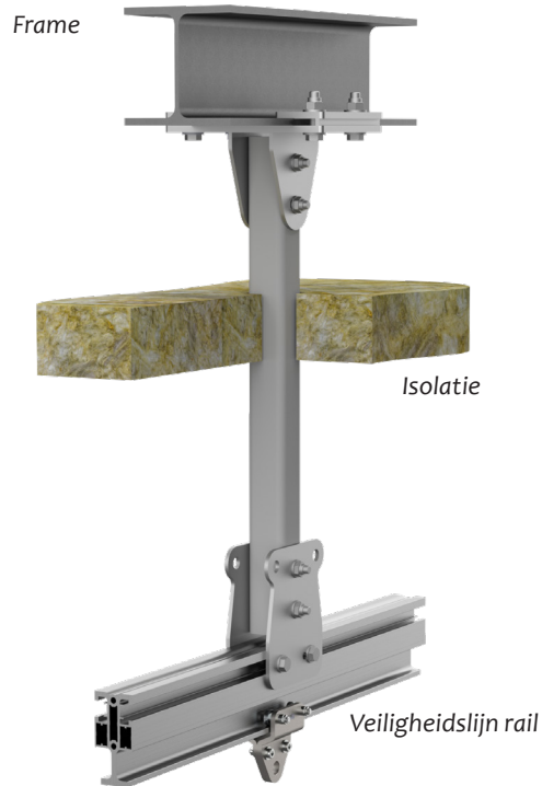
Composiet thermische isolatiekaars.
